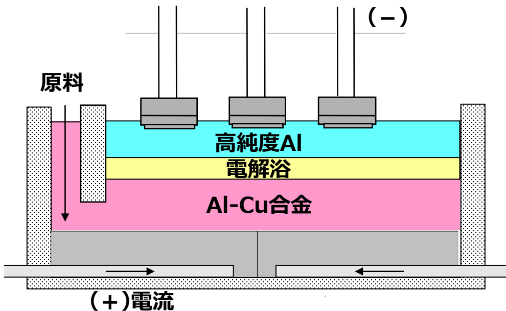
三層電解法
